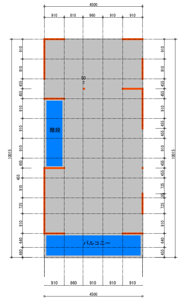
3階 柱・壁 配置図
