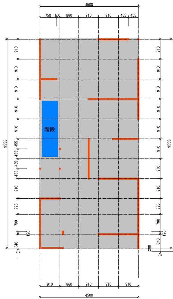
1階 柱・壁 配置図
