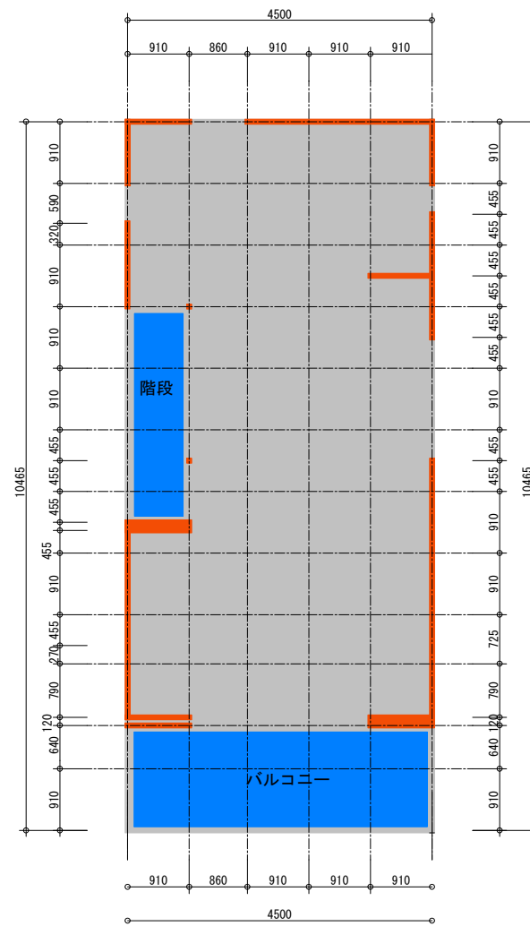
2階 柱・壁 配置図
